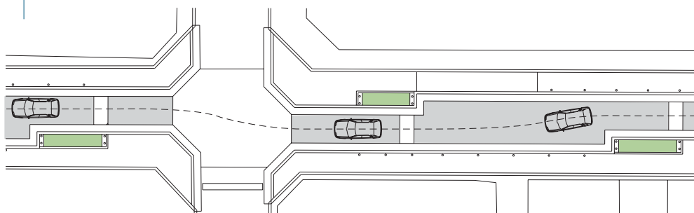
車両軌跡によるコーナー角の検討
